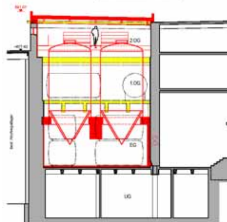
Schnitt 2-2 1:100
